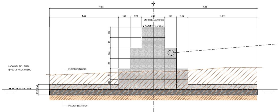
Detalle del Muro de Protección de la Margen Izquierda
