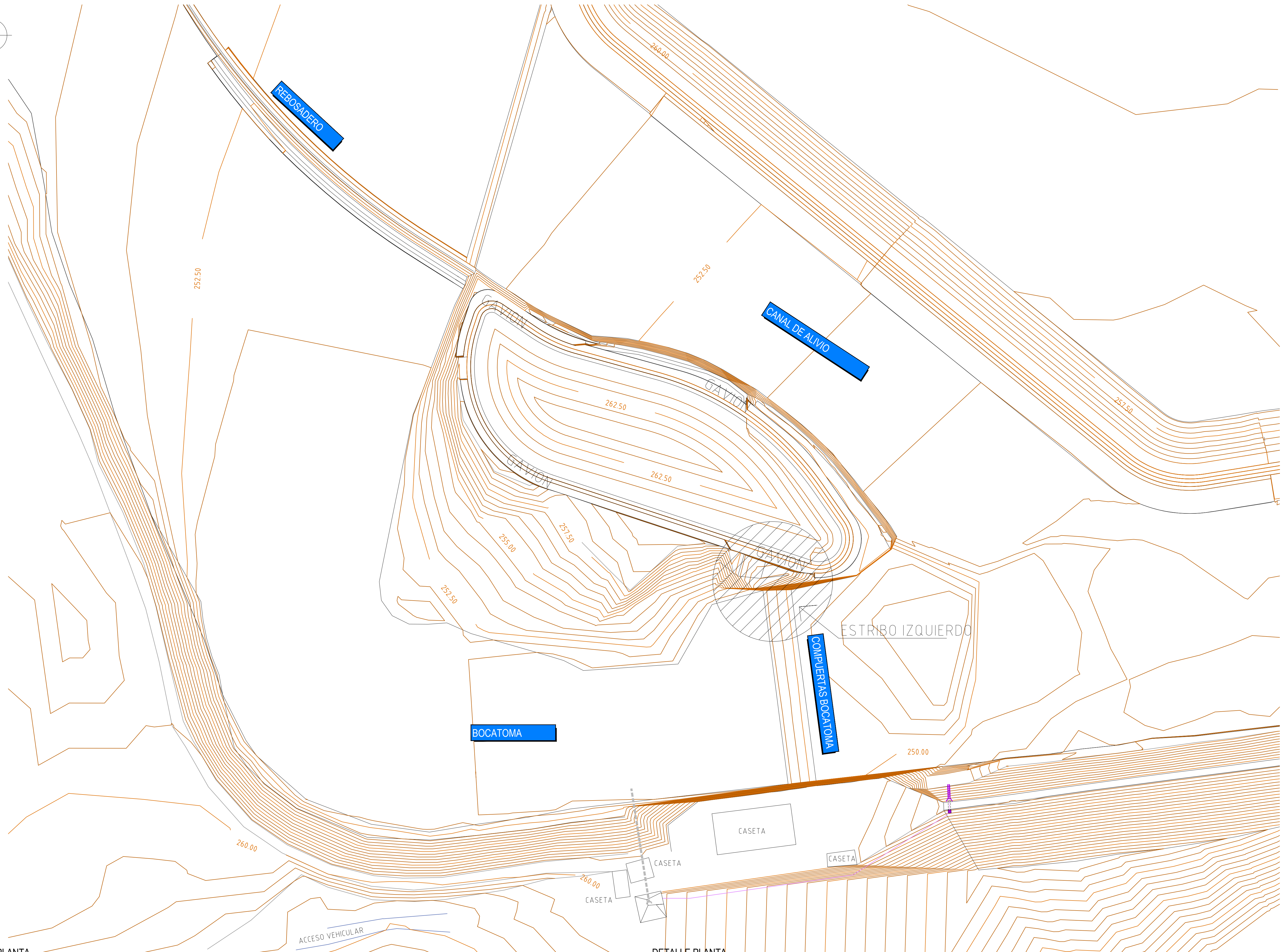
DETALLE PLANTA ESCALA 1/500
