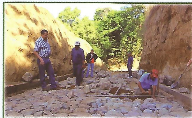
Empedrado Fraguado de Calle de acceso a Cementerio en Cantón Las Marías
