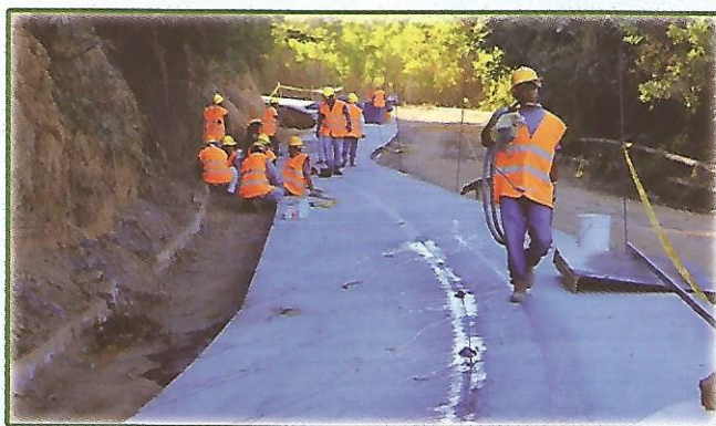
Concreteado Hidráulico de Calle de acceso a Cantón San Antonio (FUNDAGEO)
