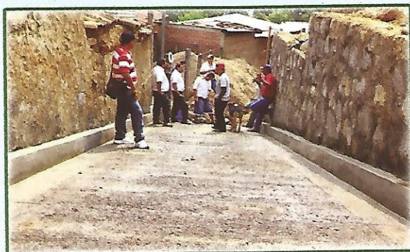
Concreteado Hidráulico de calle Final 1a Av. Sur, Barrio Yusique
