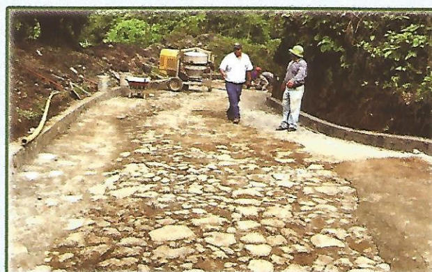
Empedrado Fraguado de calle en Cantón Copinol I
