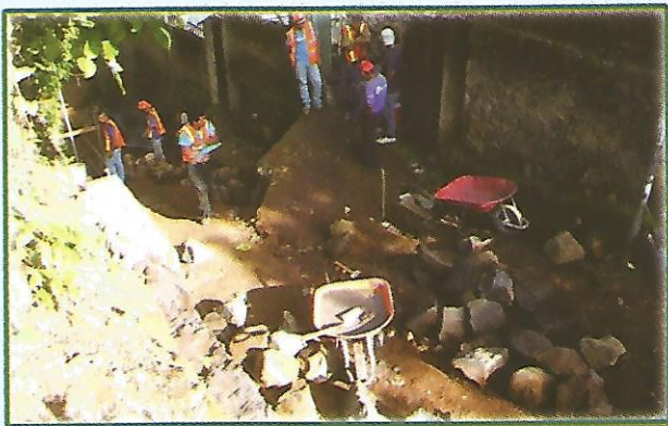
Concreto Hidráulico en calle al Final de 8° Calle Poniente, Barrio Yusique
