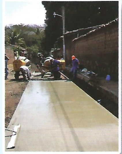
Construcción de Concreto Hidráulico en tramo de la 9° Calle Oriente sobre la Av. Nueva España, del Barrio Dolores. (100 mts. Lineales) MONTO $39,539.48
