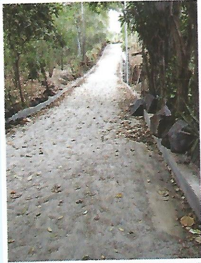
Empedrado Fraguado y cordoneado de cuesta en Calle Principal del Caserío Mama Lola, Cantón Conacastal (33 mts. Lineales)
