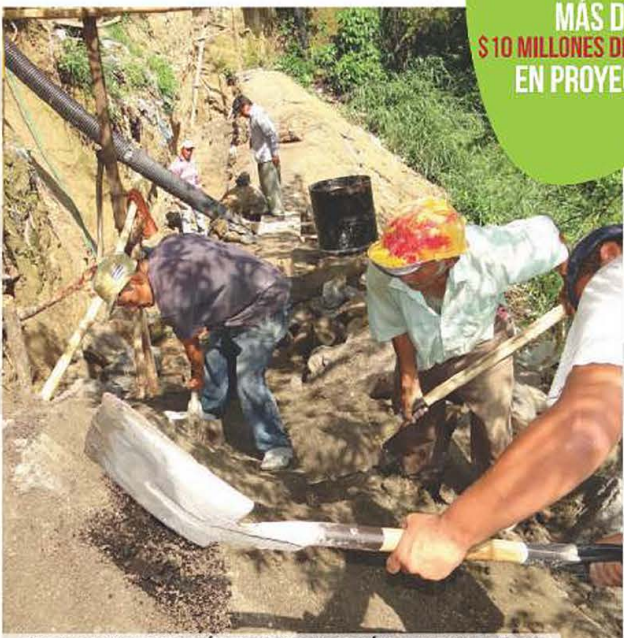
MURO DE CONTENCIÓN EN LOTIFICACIÓN CAMPO AMOR 2
