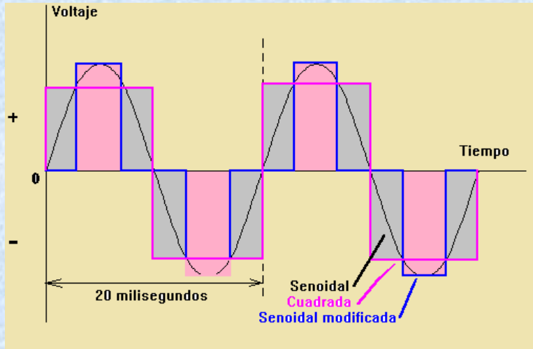
ONDA SINOSOIDAL PURA DE REFERENCIA
