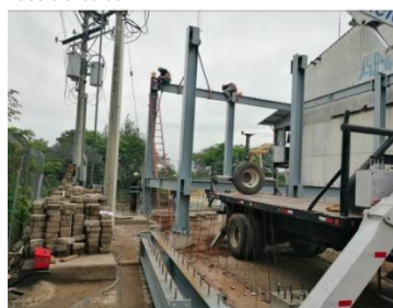
NUEVA SALA ELECTRICA. Colado de las fundaciones para la nueva sala eléctrica e Instalación de perfilera de acero
