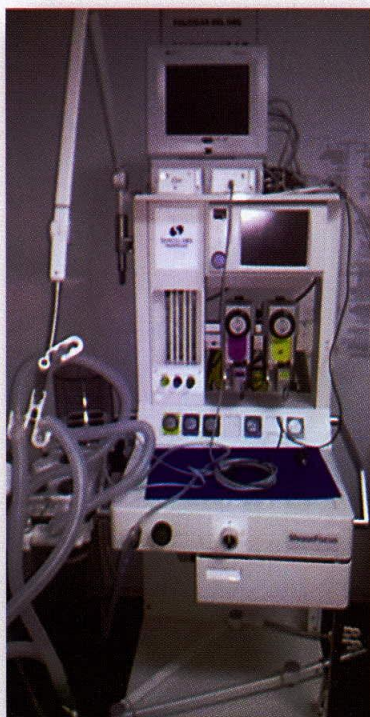
Tres (03) Maquinas de Anestesia con Capnografía
