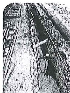
Colocación de suelo cemento para anclar tubería por presencia de agua en frente 6
