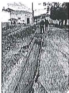
Compactación de zanja en la cual se ha colocado tubería en Frente 6
