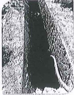
Drenado de agua en zanja en sector de frente 6
