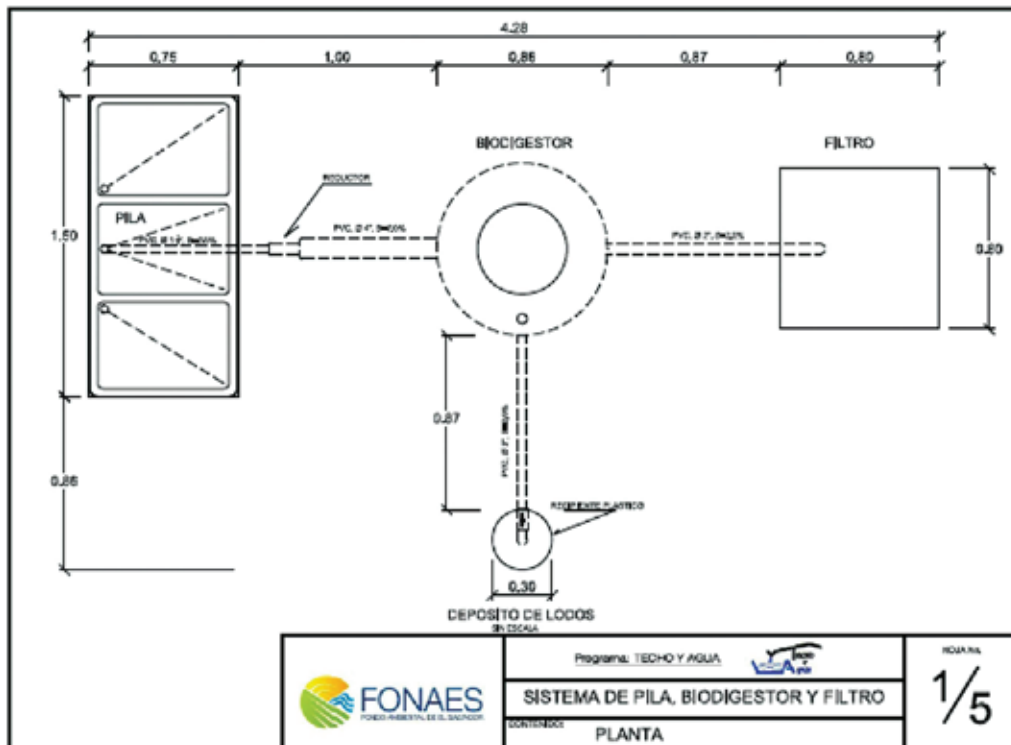
Plano general del sistema de Saneamiento Básico que incluye el sistema de biodigestor y lavaderos.
