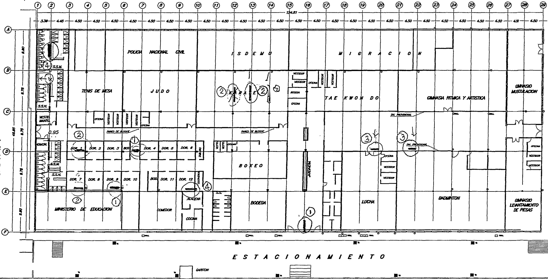
PLANTA ARQUITECTONICA EXISTENTE. ESCALA 1:250.
