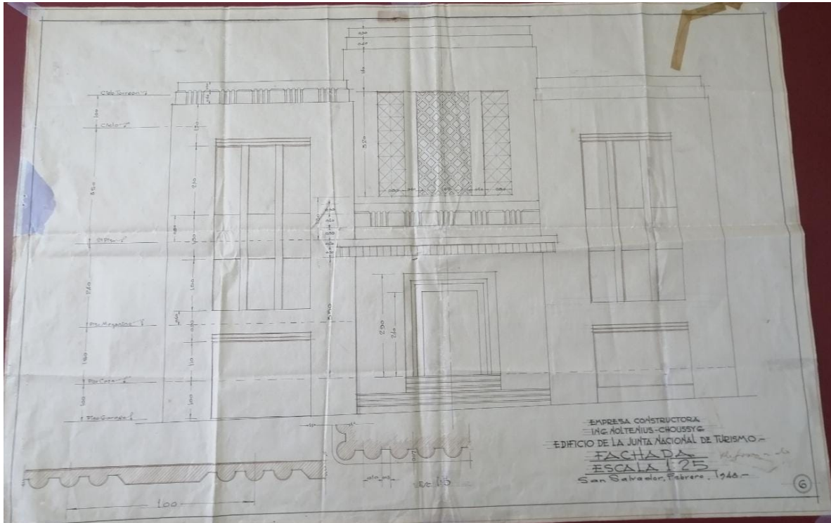
8-PLANO EDIFICIO ISTU-DARIO
