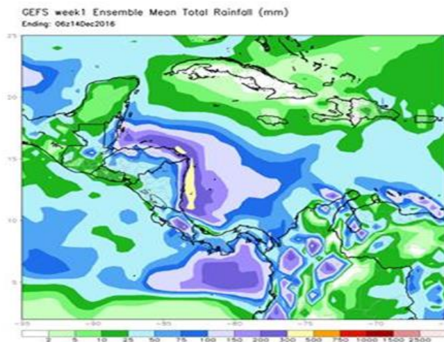
Figura 1: Pronóstico de una semana de lluvia total.
