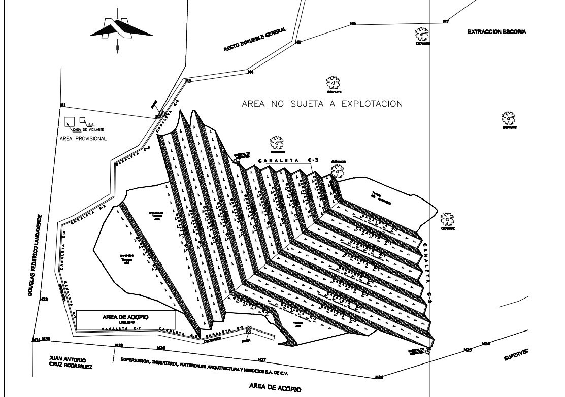
PLANO GENERAL DE DE UBICACION Y PERFILES DE OBRAS HIDRAULICAS ESC. 1 : 750
