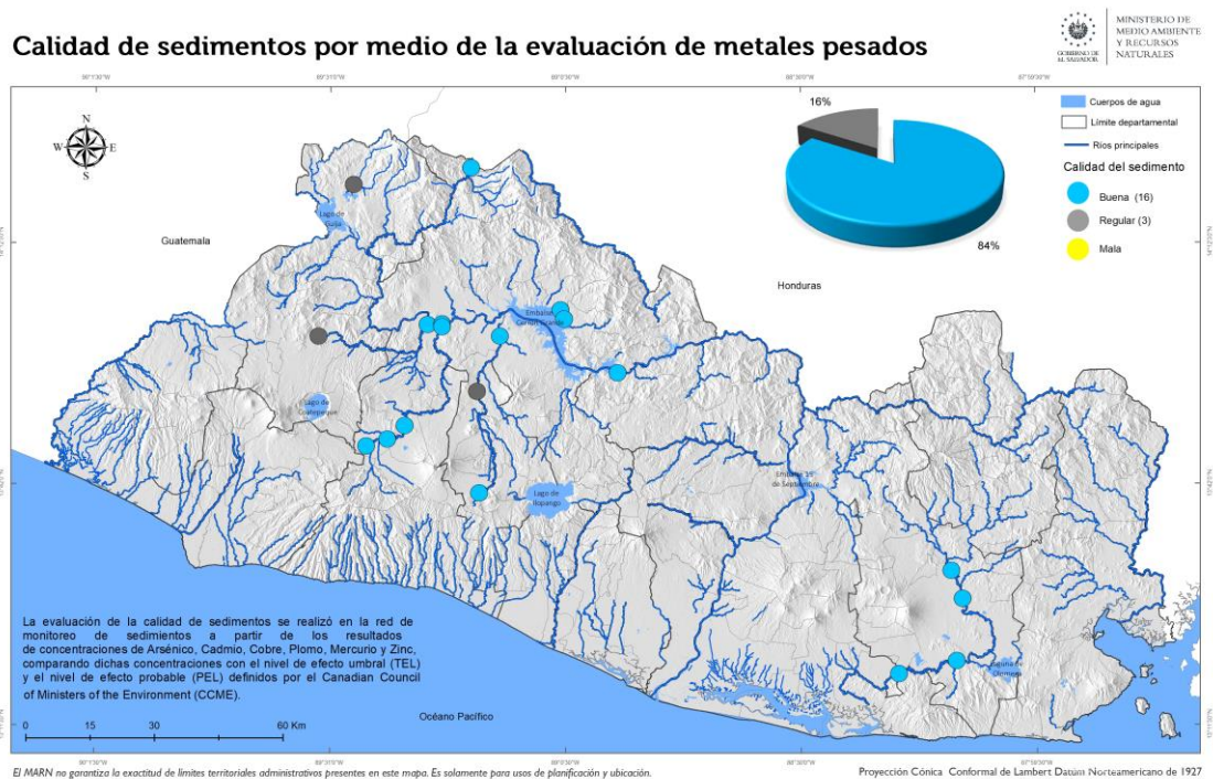
Figura 13. Resultados de la calidad de sedimentos del país Fuente: MARN
