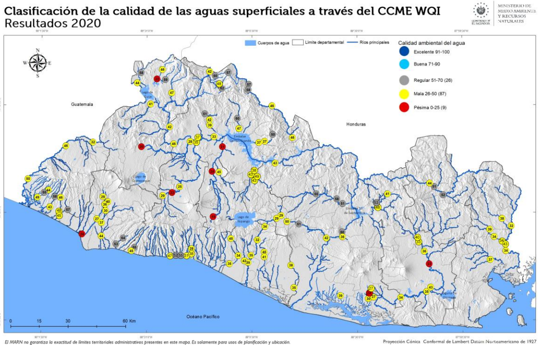
Figura 6. Calidad de agua valorada a través del Índice de Calidad de Agua (CCME — WQI), para el año 2020.
