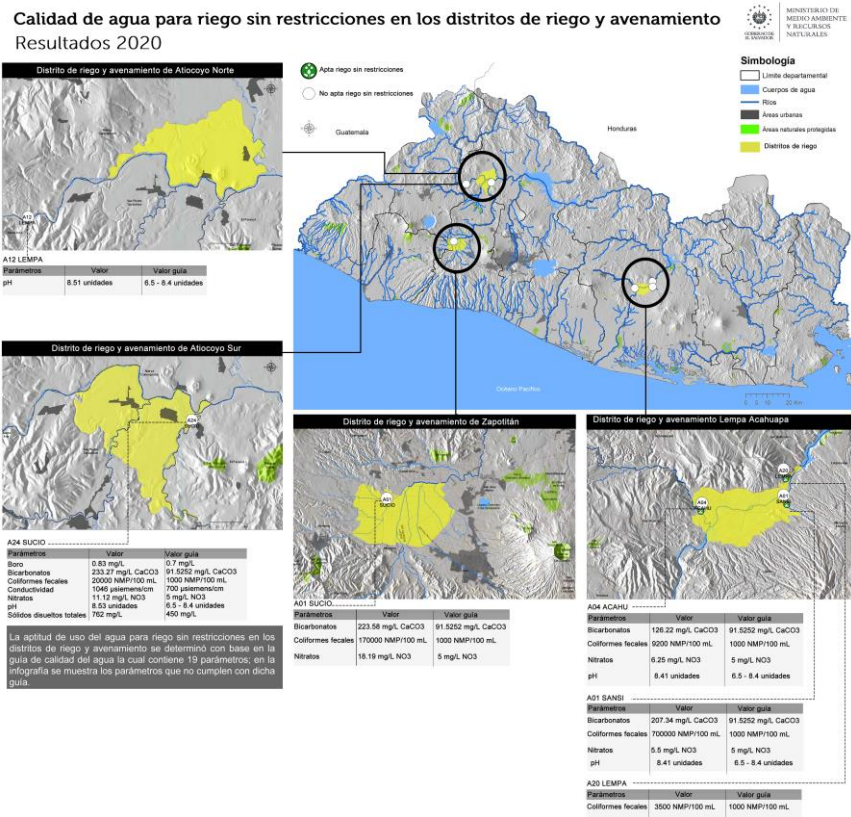
Figura 10. Resultados de calidad de agua para riego sin restricciones en los distritos de riego y avenamiento Fuente: MARN
