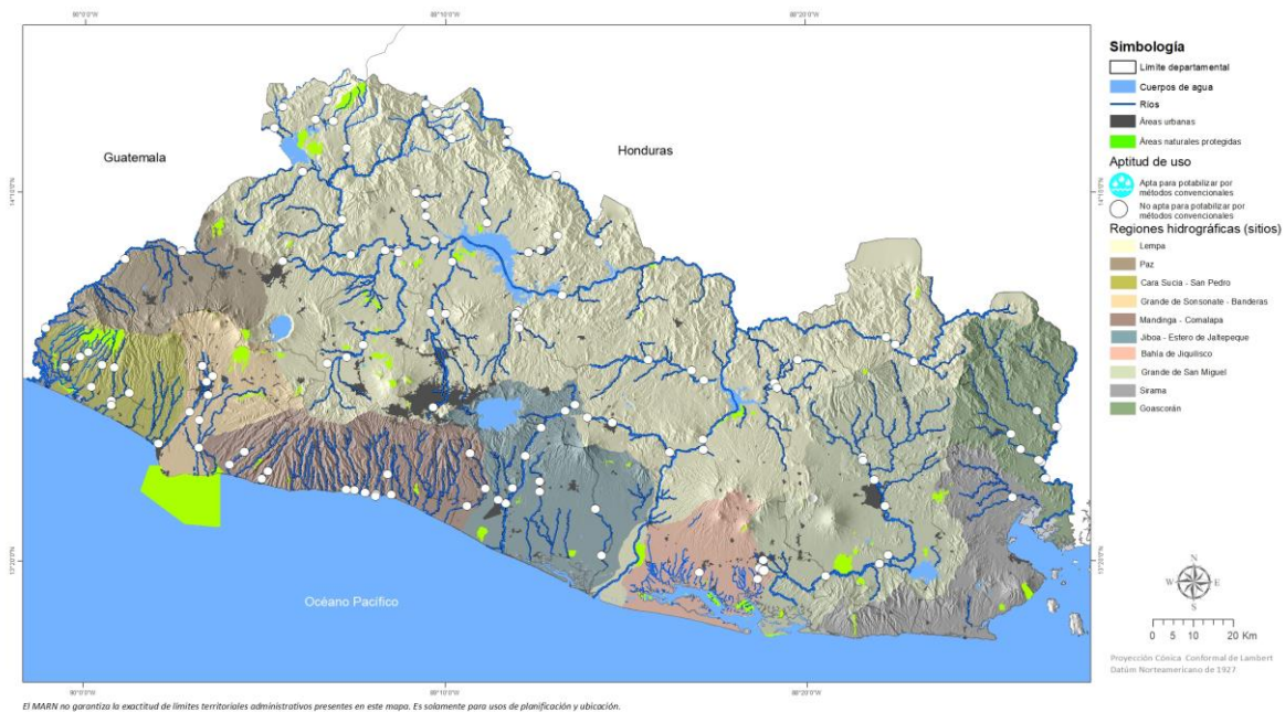
Figura 8. Resultados de calidad de agua para potabilizar por métodos convencionales. Fuente: MARN.
