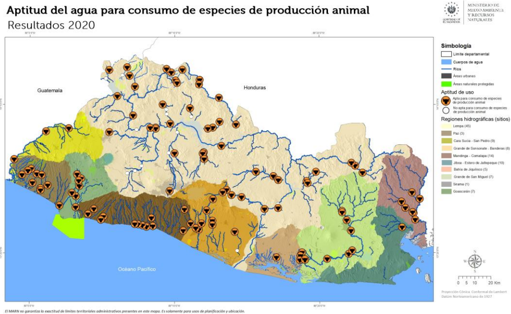
Figura 11. Resultados de calidad de agua para consumo de especies de producción animal. Fuente: MARN.
