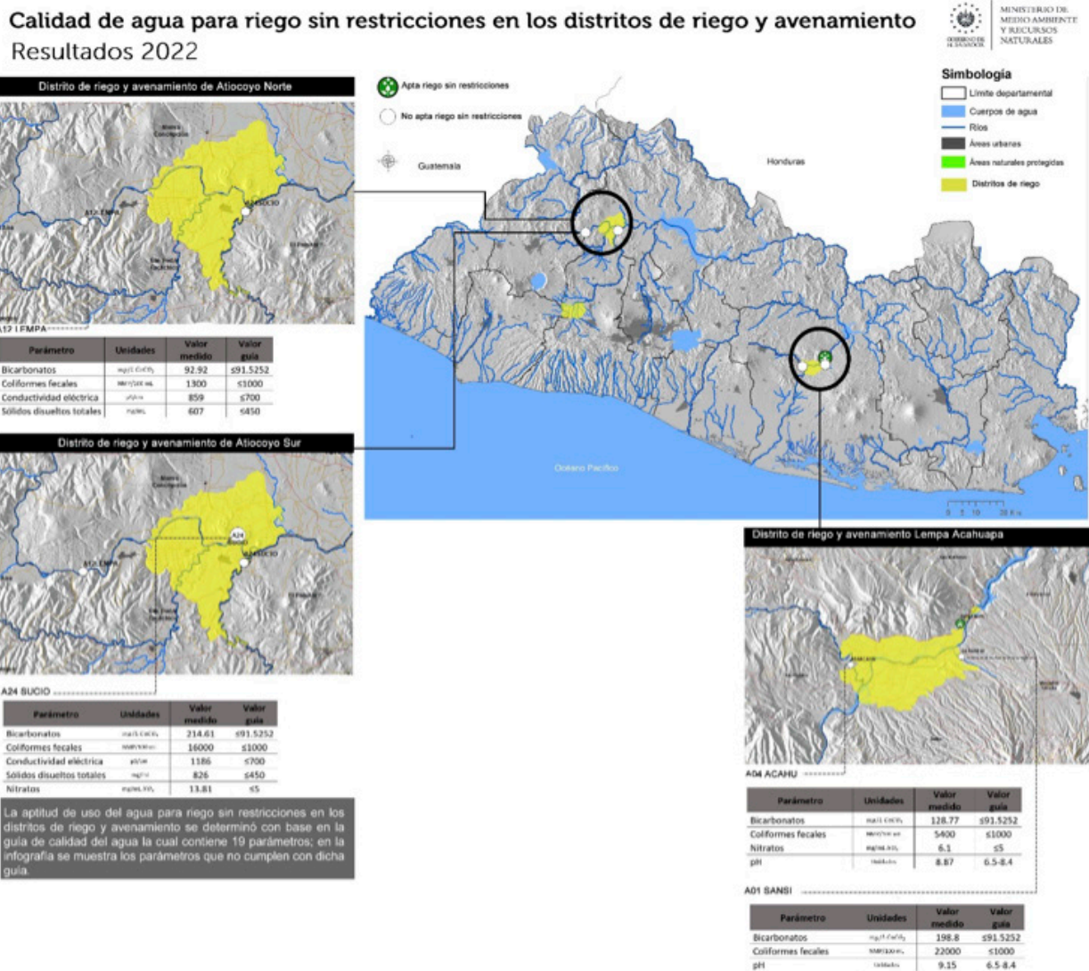
Figura 8 Resultados de calidad de agua para riego sin restricciones en los distritos de riego y avenamiento. Fuente: Ministerio de Medio Ambiente
