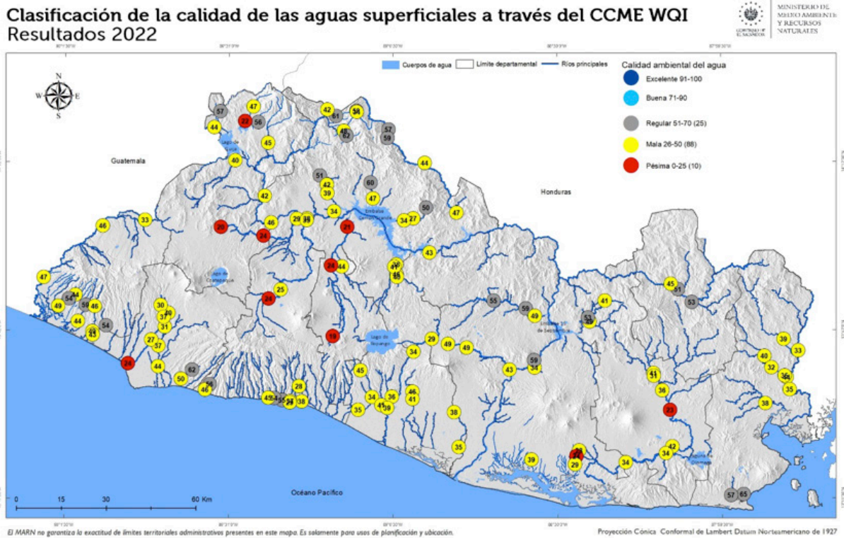
Figura 4 Calidad de agua valorada a través del Índice de Calidad de Agua (CCME – WQI), para el año 2022.
