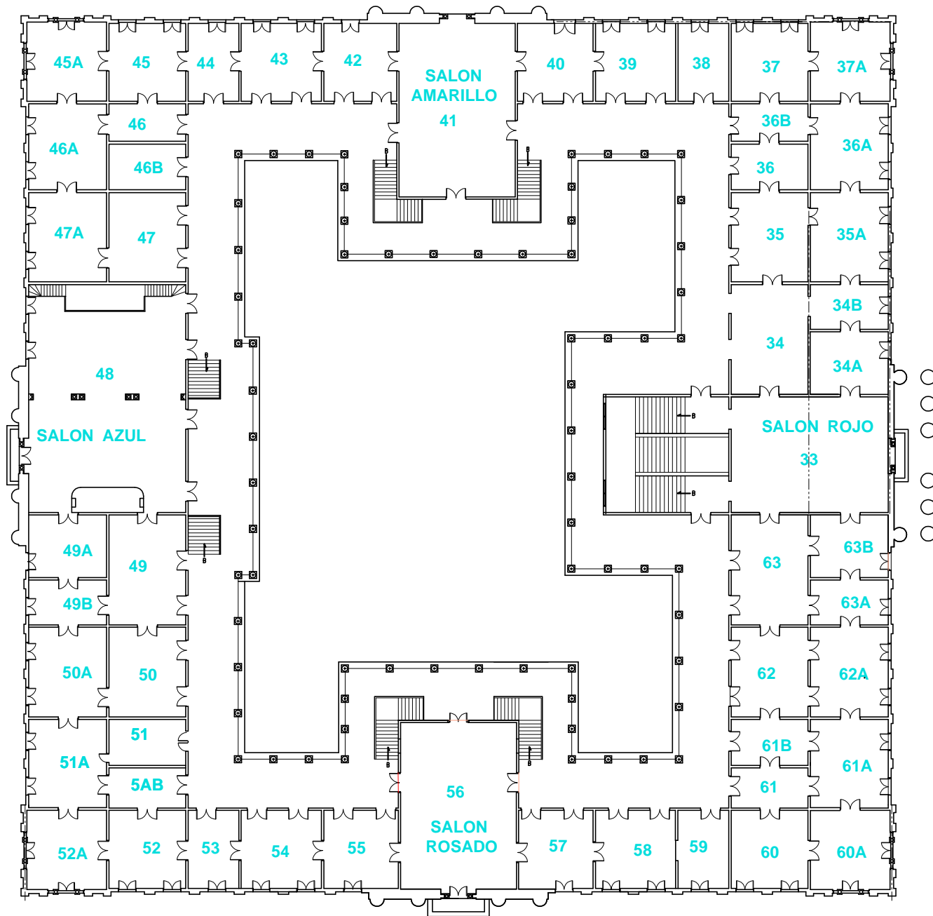
PLANTA ARQUITECTONICA 2do NIVEL PALACIO NACIONAL SIN ESCALA
