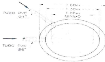
PLANTA DE POZO DE ABSORCION ESCALA 1 : 5 0
