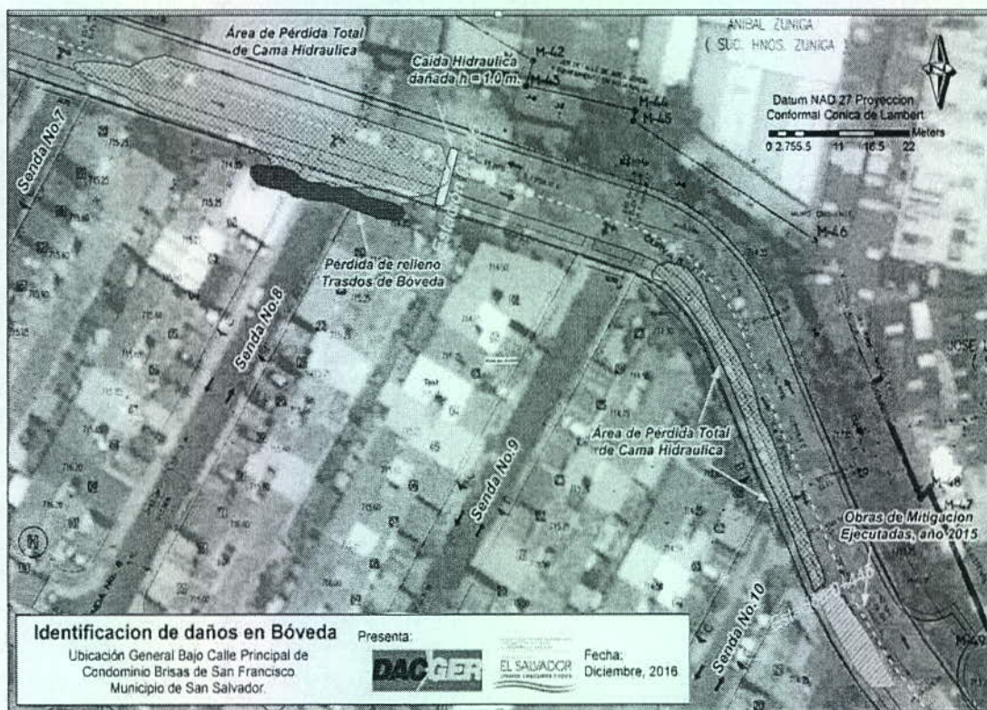
Figura 2. Esquema de ubicación específico
