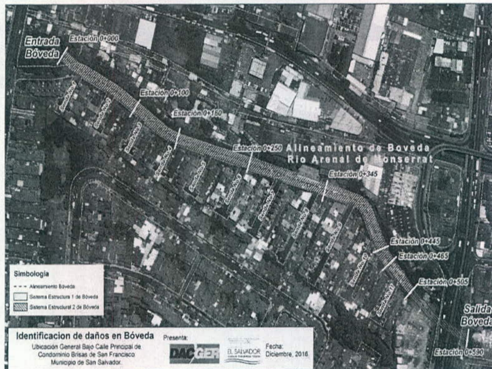
Figura 1. Esquema de ubicación general
