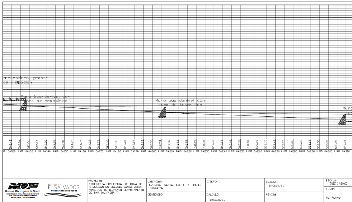
Figura 3. Esquema de obra propuesta de muros guardanivel en perfil.
