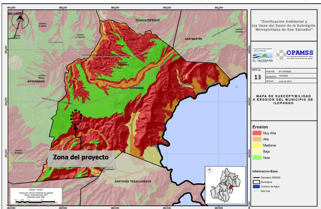
MAPA No. 2. El proyecto en el mapa Geomorfológico del municipio de Ilopango.
