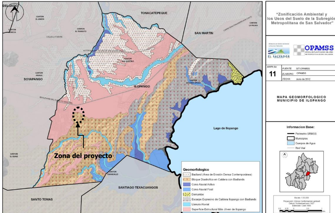
MAPA No. 1. Tipos de rocas existentes en la zona del proyecto.
