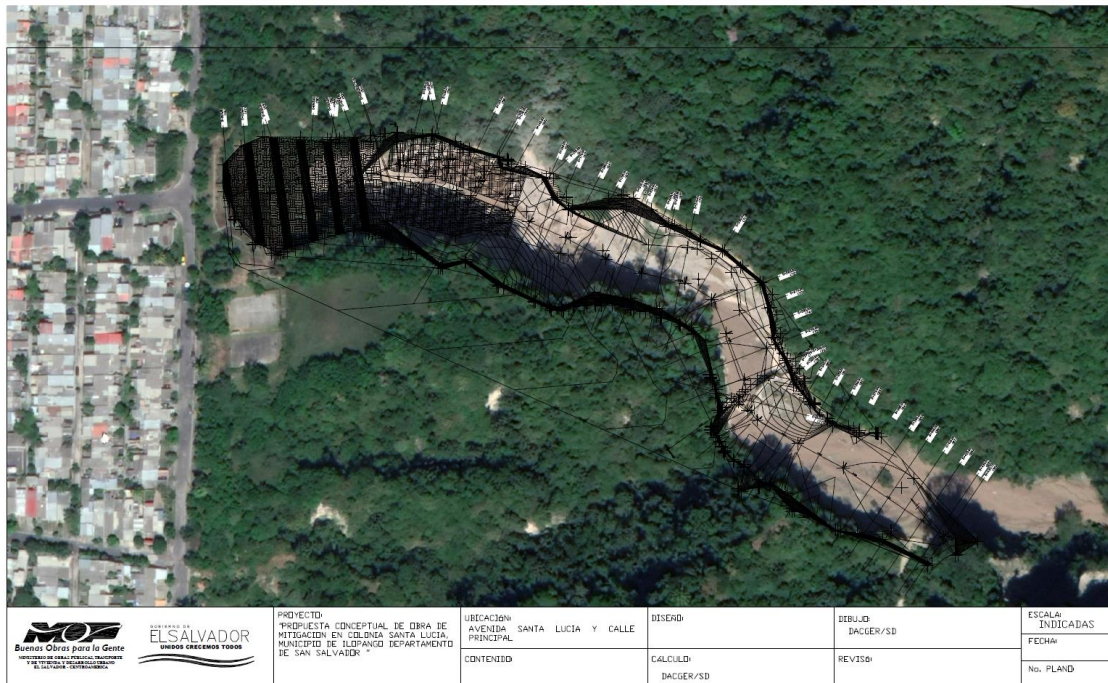
Figura 5. Planta del alineamiento considerado para la cárcava Santa Lucía. El área achurada detalla la intervención dentro de los límites de la cárcava y el cauce de la quebrada.
