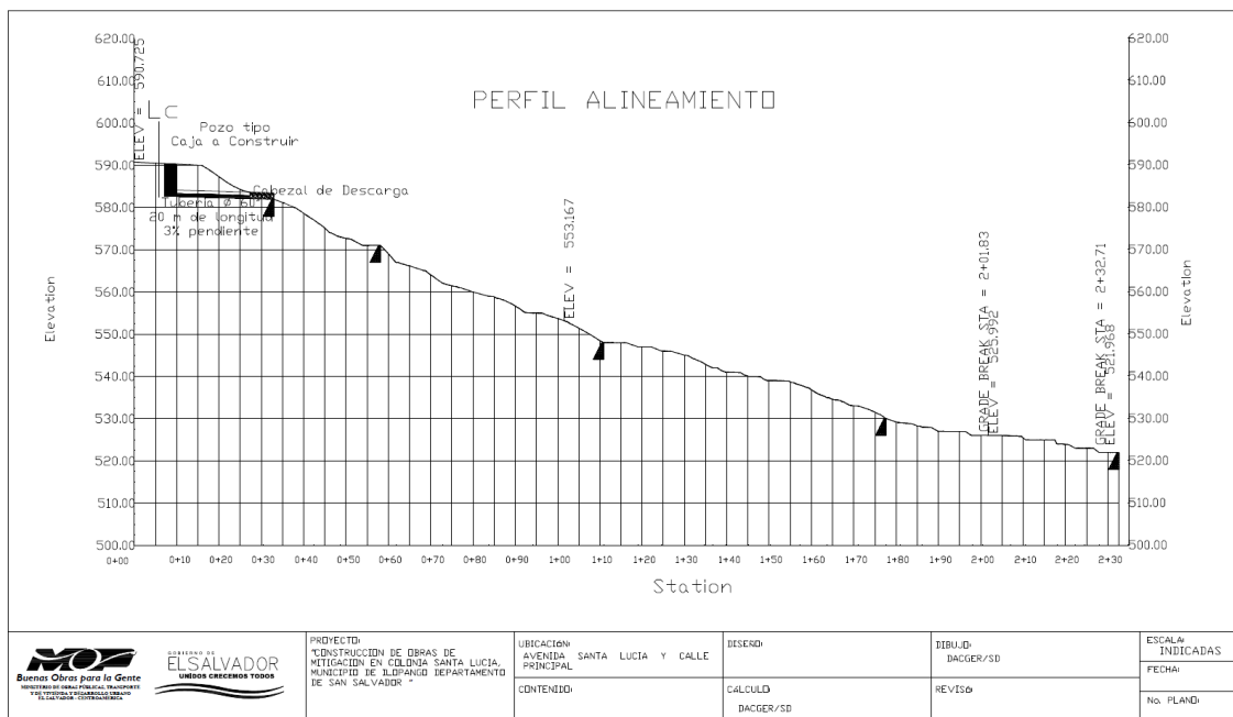
Figura 1. Obras en el sector donde se desviarán las aguas lluvias que comprende: pozo, 20 m de tubería, cabezal de descarga y muros guardanivel.
