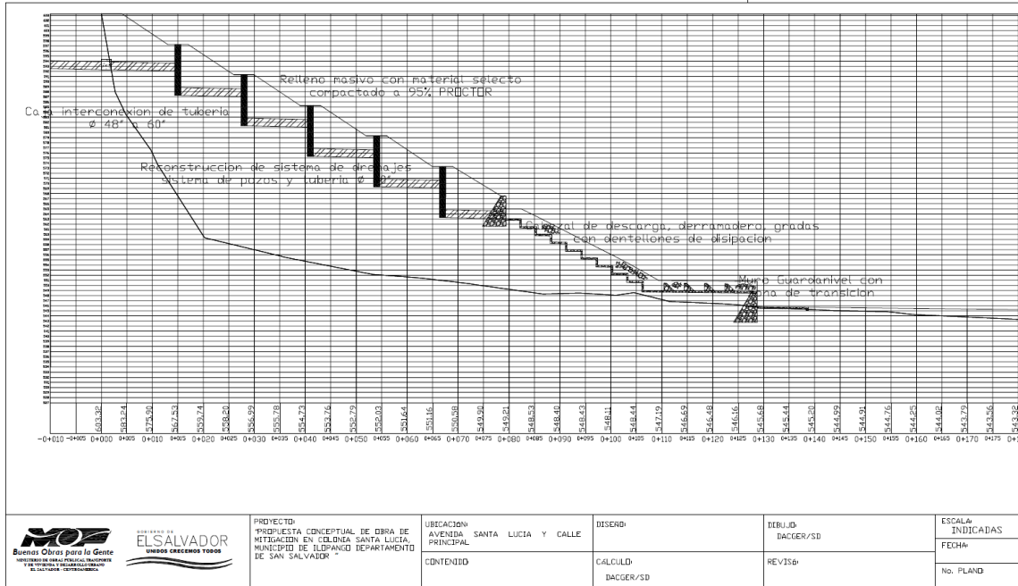
Figura 2. Esquema de obra propuesta, Vista de Perfil.
