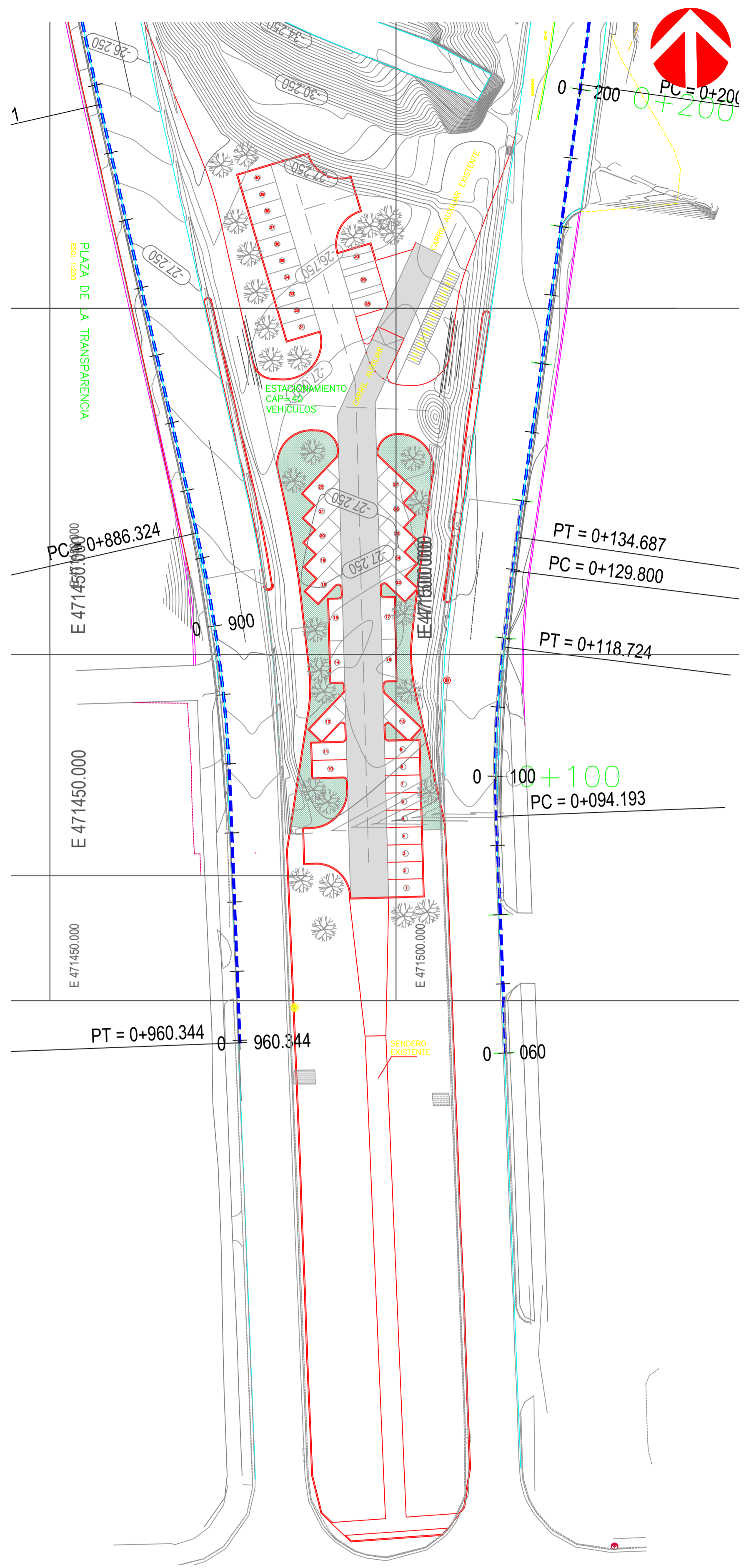
PLANTA DE CONJUNTO ESC. 1:1000
