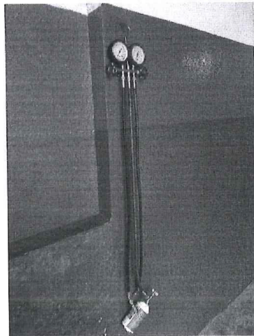
PROBADOR DE FUGAS DE SISTEMA DE REFRIGERANTES
