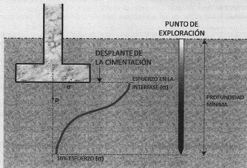
Figura 0.2 Profundidad respecto al incremento de esfuerzo
