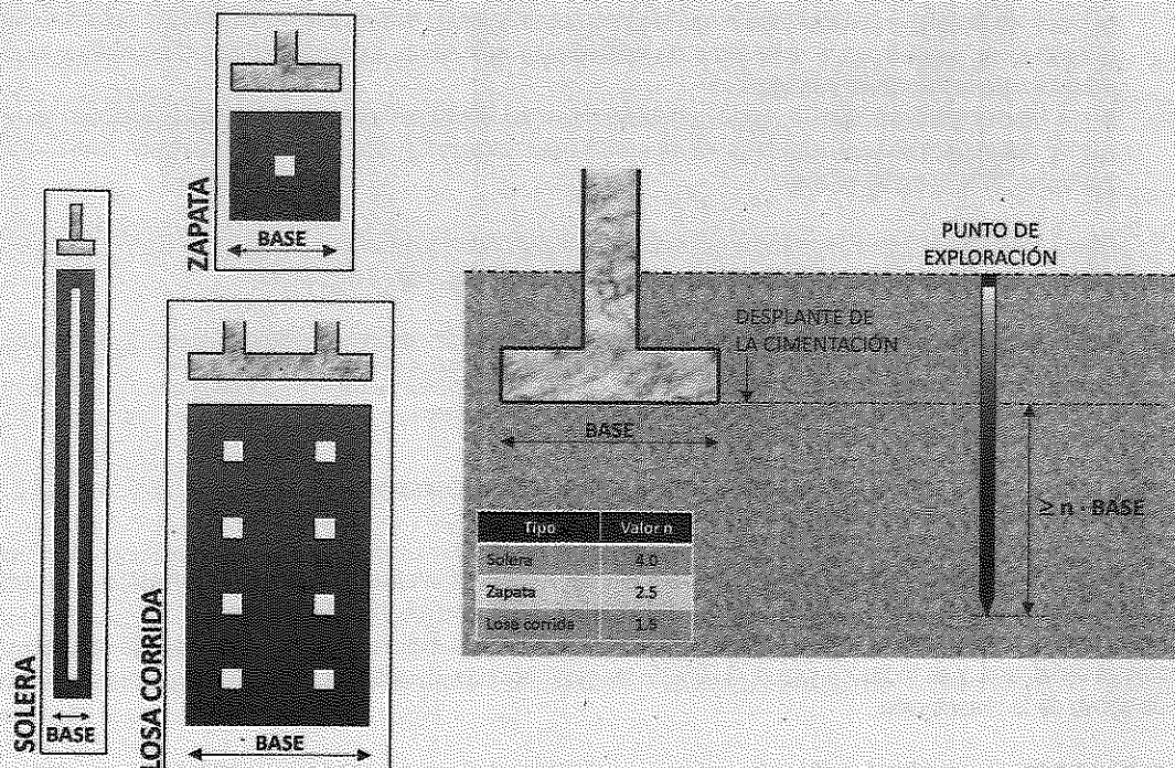
Figura 0.3 Profundidad respecto cimentaciones superficiales
