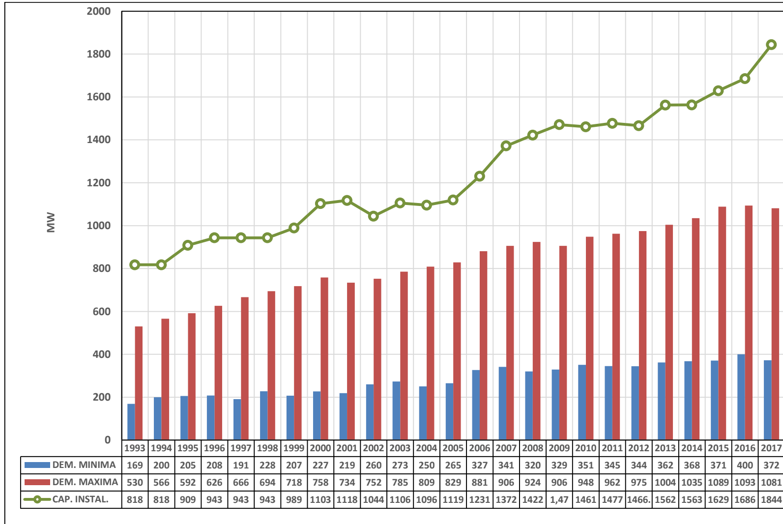
GRÁFICA 18: CAPACIDAD INSTALADA, DEMANDA MÁXIMA Y MÍNIMA (1993 - 2017)
