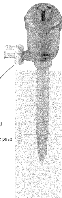
EK226SU roscado, con llave de paso 110 mm
